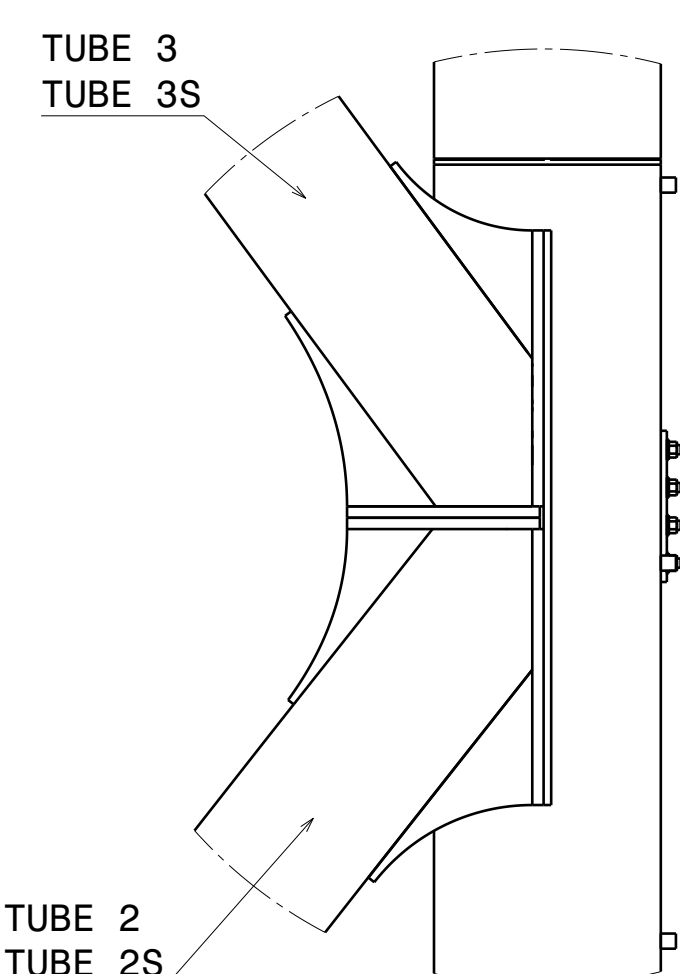
N12 Scale: 1:10
