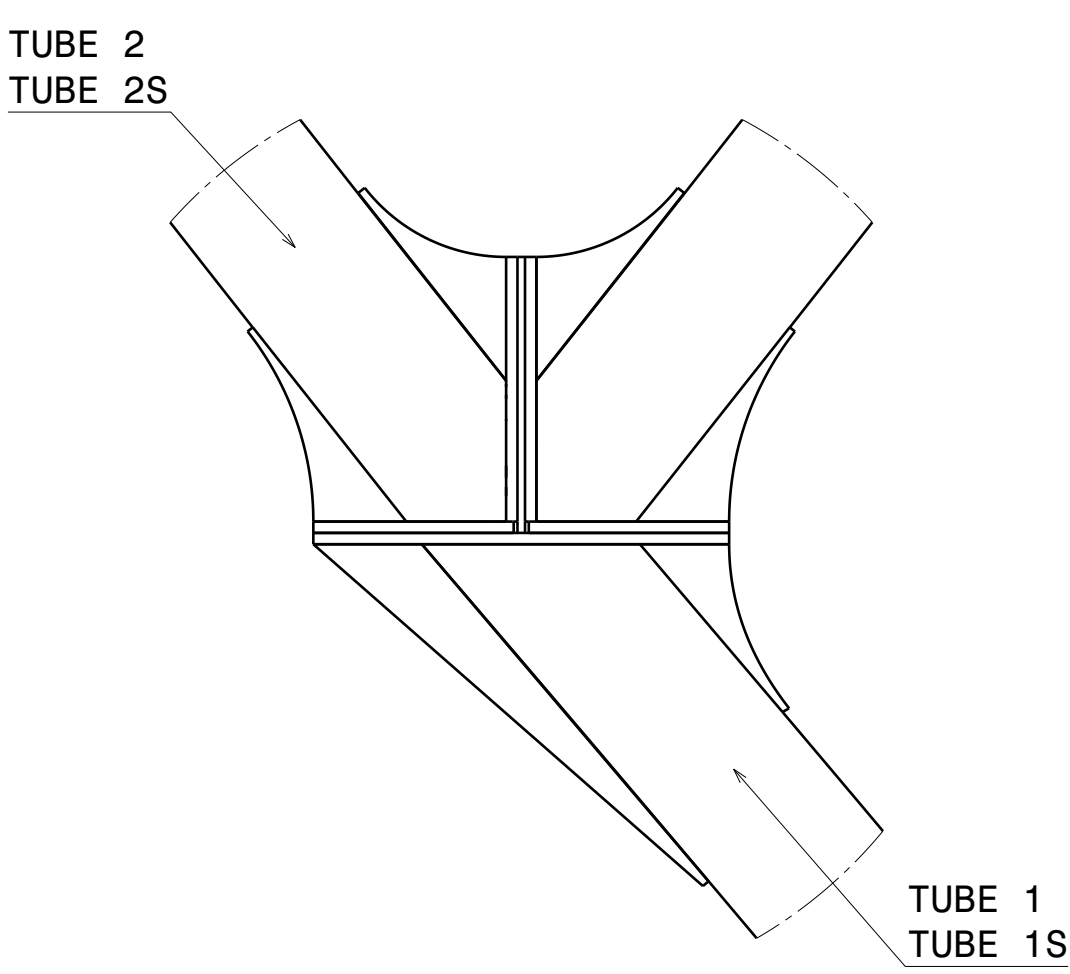
N11 Scale: 1:10
