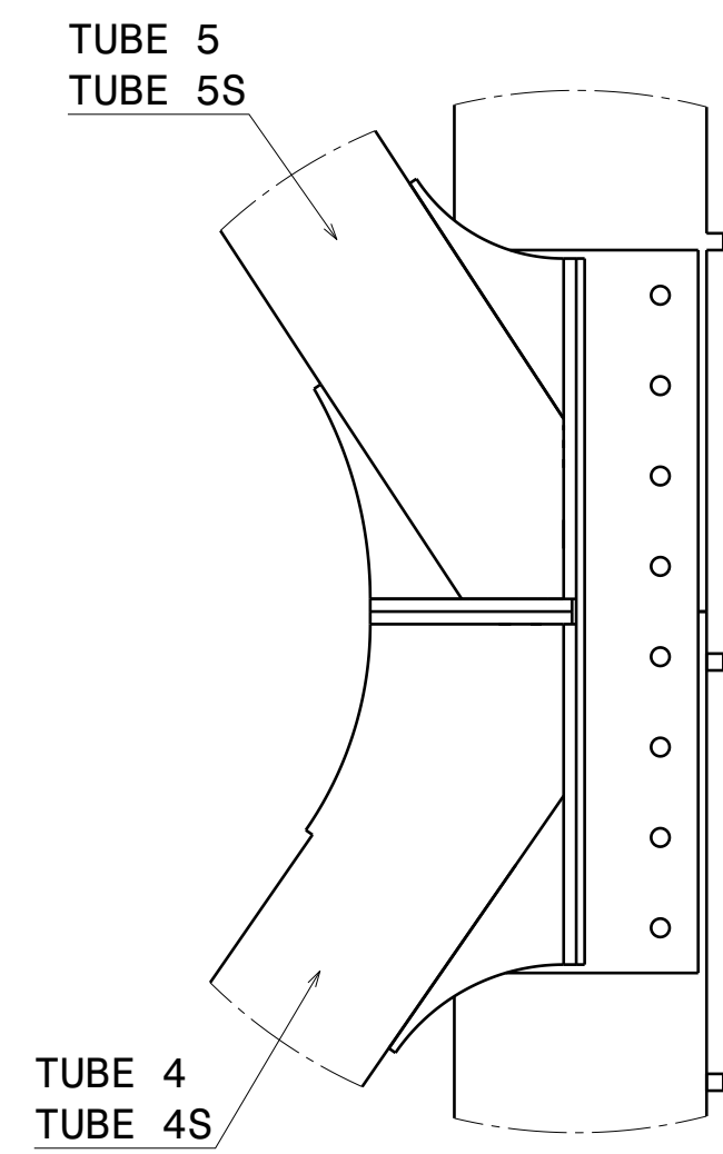
N15 Scale: 1:10
