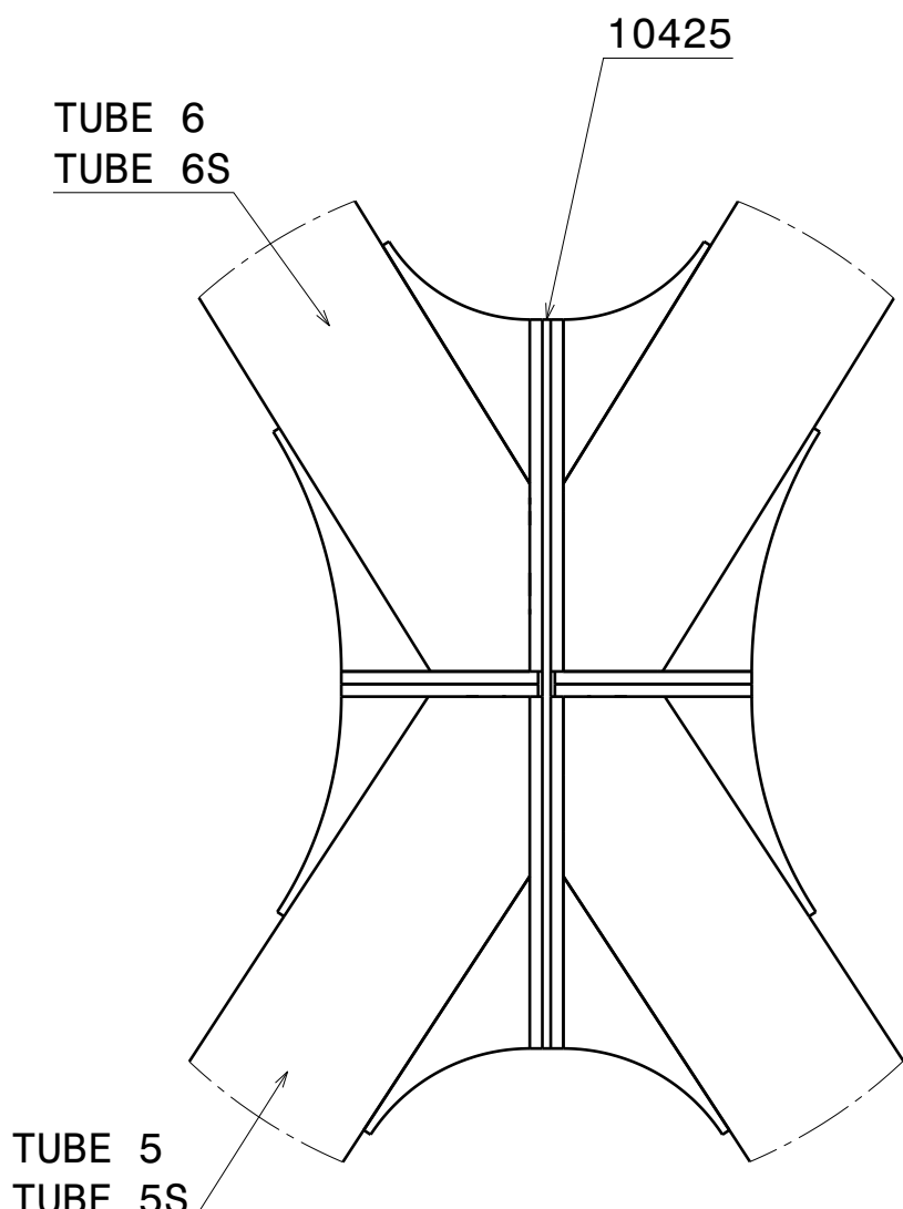
N17 Scale: 1:10
