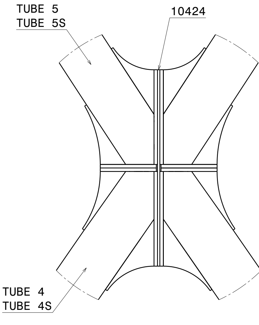
N16 Scale: 1:10
