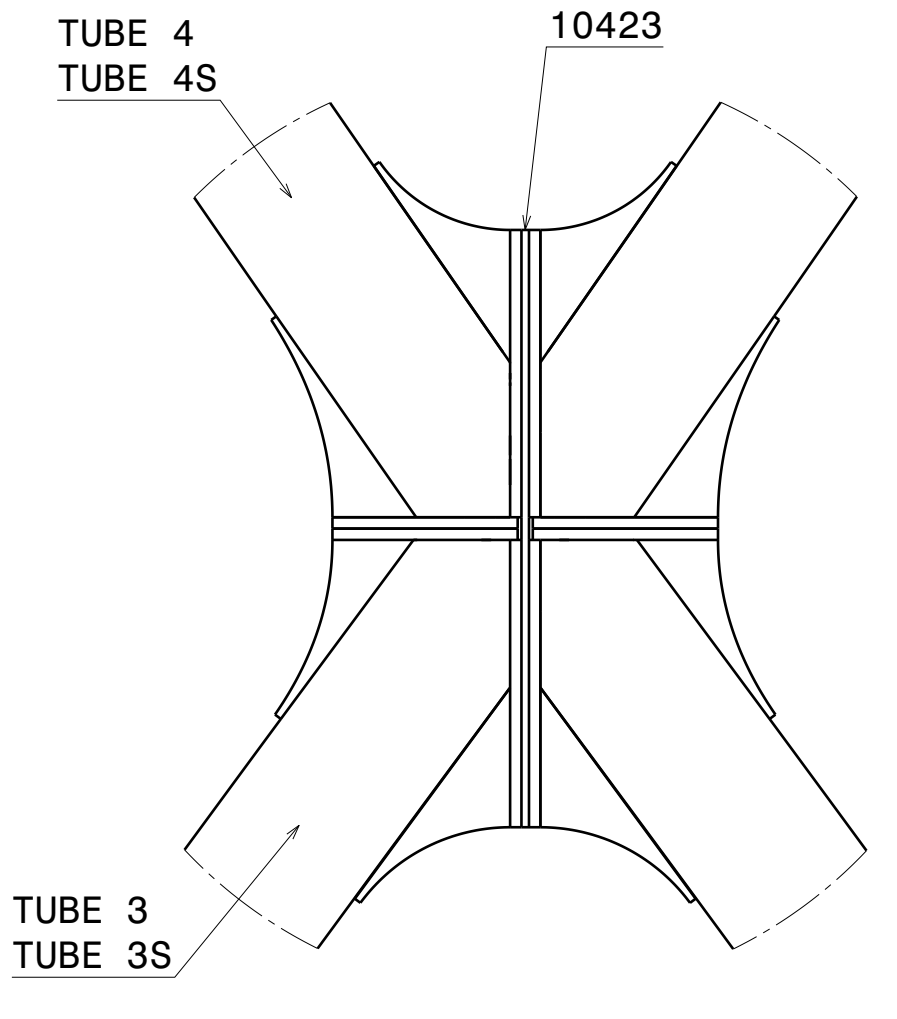
N14 Scale: 1:10
